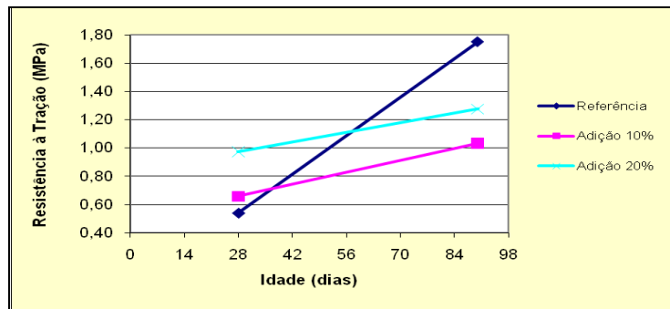
Figura 06 – Ensaio de Resistência à Tração
